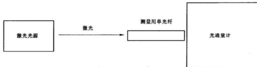
图 A.2 出射光的测量装置
